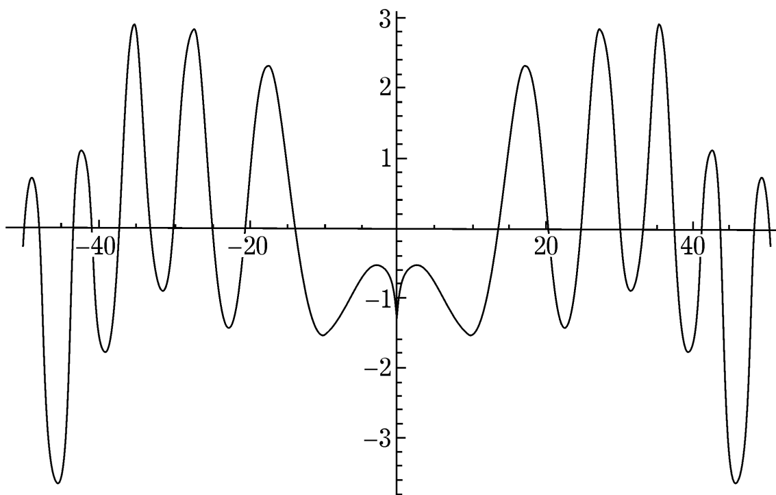
График \xi\left(\frac{1}{2} + it\right) , -50 < t < 50
